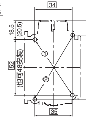
安装孔尺寸图
