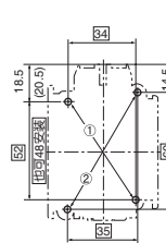
安装孔尺寸图
