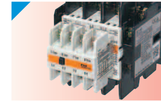
辅助触头单元(顶部安装) (SZ-A□型) 该单元是在所有触头上采用了双触头的2触头及4触头的辅助触头单元,可快速安装于电磁接触器。
