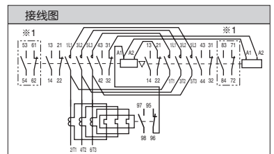
※1 辅助触头3NO + 3NC × 2时 ※2 控制电路电源用M4螺孔
