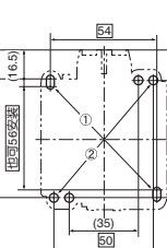
安装孔尺寸图
