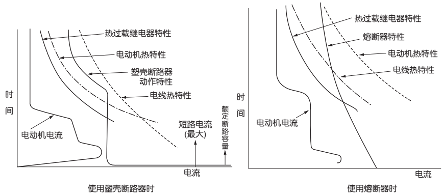
电动机电路中的保护协调特性曲线
