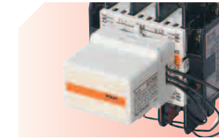
主电路电涌吸收单元 (顶部安装、侧面安装)(SZ-ZM□型) 内置三相电动机的开关电涌吸收用CR元件。
