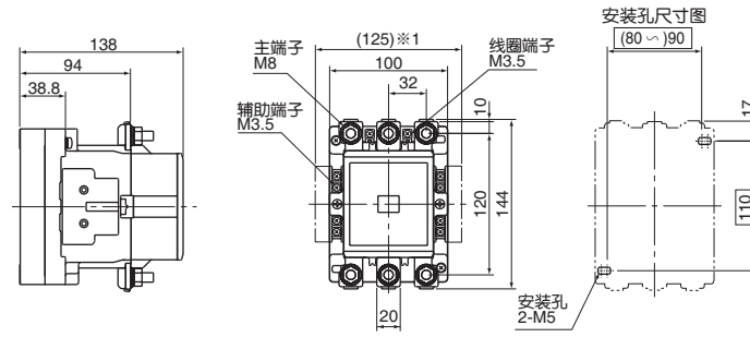
※1 侧面安装2个辅助触头单元时
