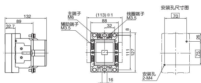
※1 侧面安装2个辅助触头单元时
