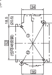
安装孔尺寸图
