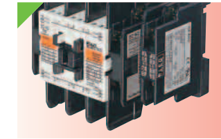
辅助触头单元(侧面安装) (SZ-AS□型) 该单元是采用了高可靠性辅助触头的2触头(1a1b)辅助触头单元,可快速安装于电磁接触器。
