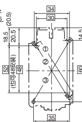
安装孔尺寸图
