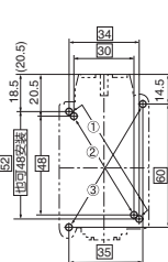
安装孔尺寸图
