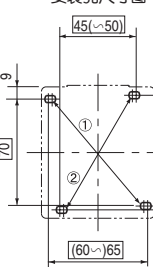
安装孔尺寸图
