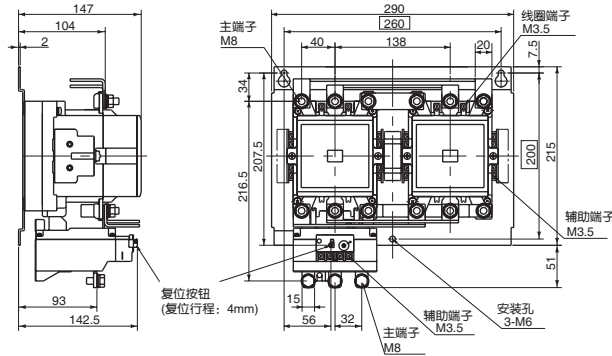
※1 辅助触头3NO + 3NC × 2时
