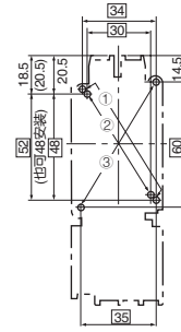
安装孔尺寸图
