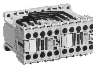
SC-M01RM/G型 (照片No.AF00-69)
