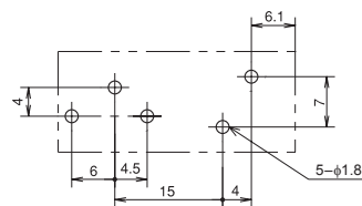
印刷板加工图(BOTTOM VIEW)
