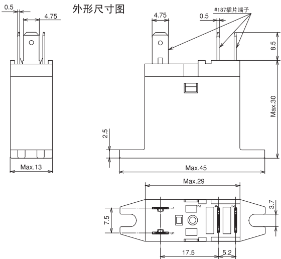
外形尺寸图
