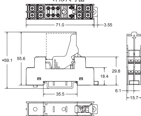
外形尺寸图
