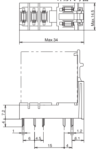
外形尺寸图
