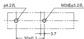
安装孔加工图
