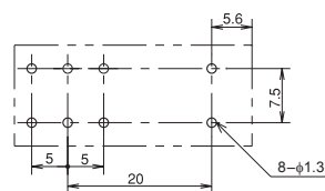
印刷板加工图 (BOTTOM VIEW)
