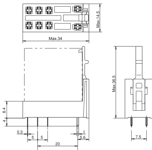
外形尺寸图
