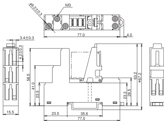
外形尺寸图
