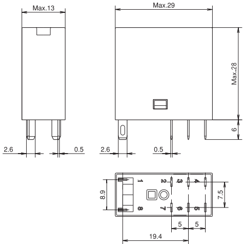
外形尺寸图
