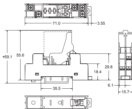
外形尺寸图
