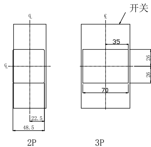
面板开孔尺寸
