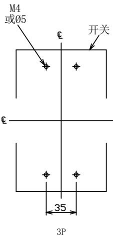
钻孔图
