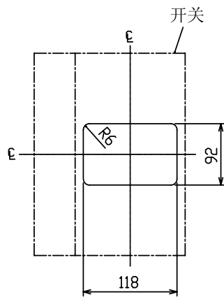
面板孔尺寸图
