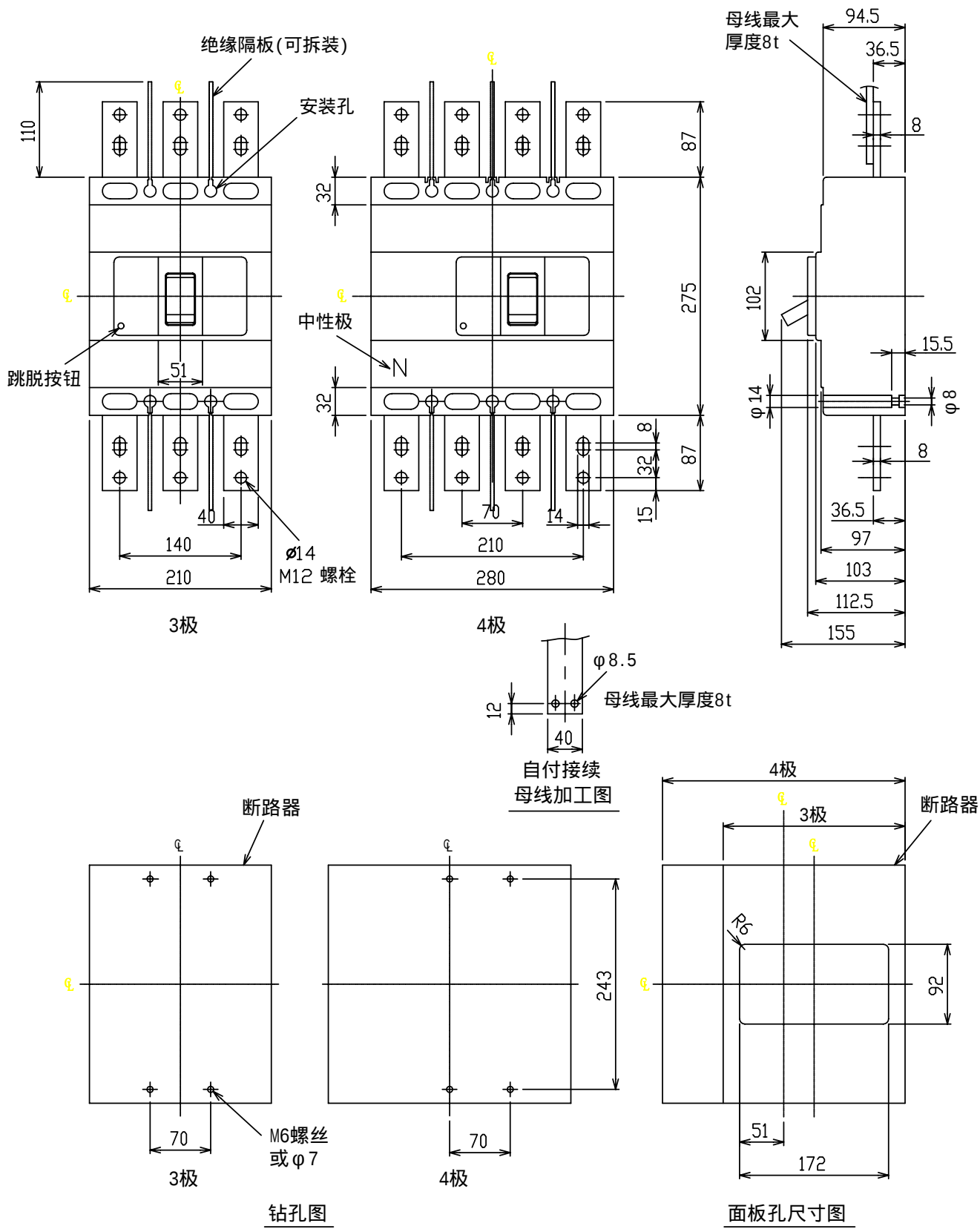
BM630-SN, HN, RN, UN 外形及安装尺寸图
