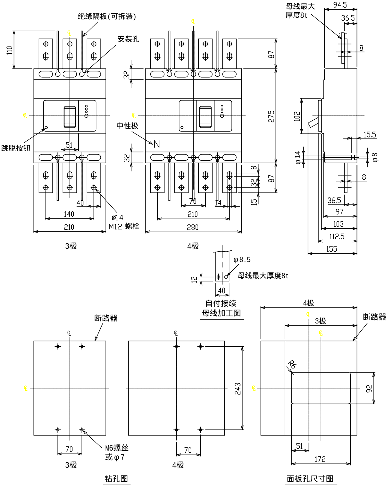
BL630-HN,RN,UN 外形及安装尺寸图
