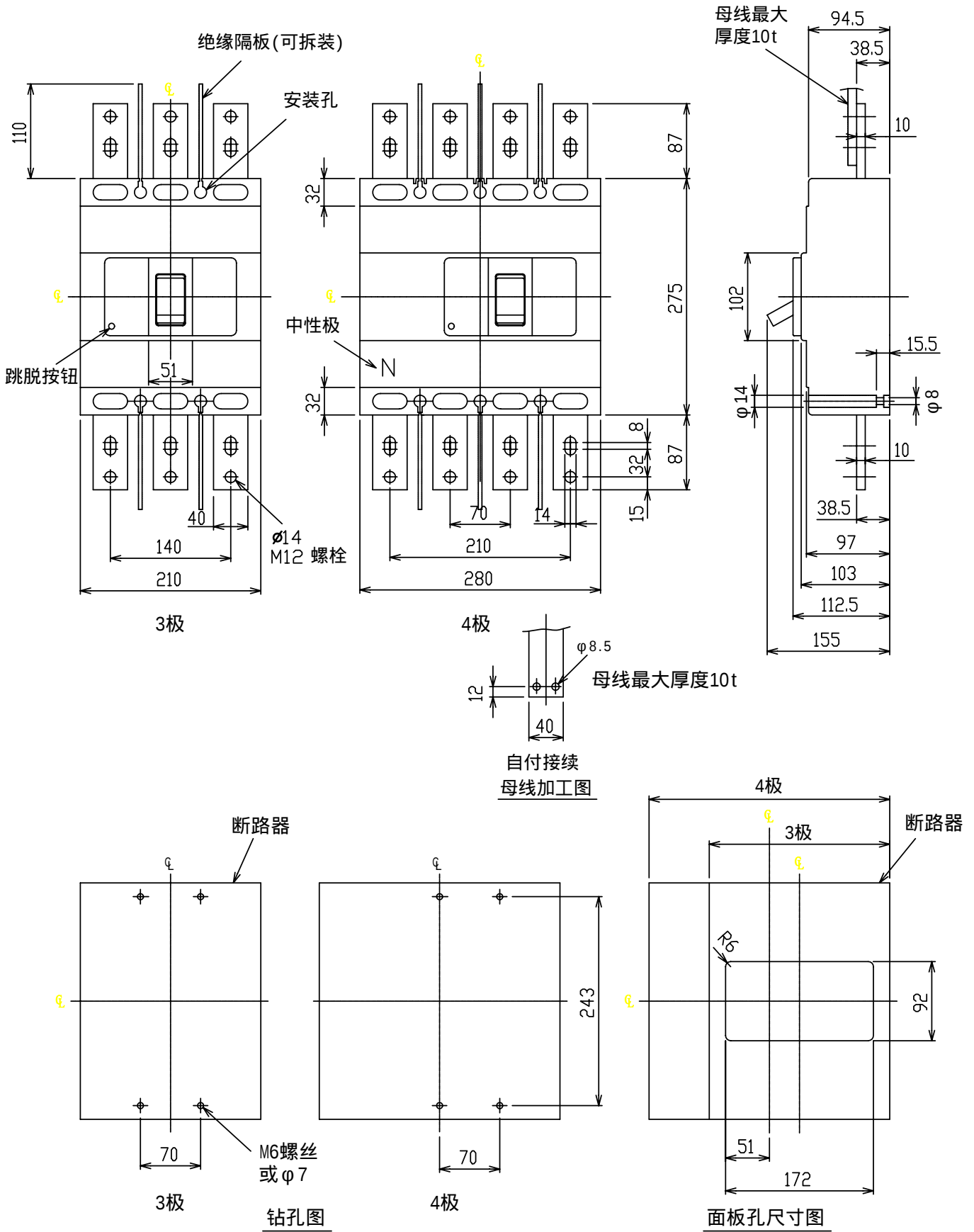
BM800-CN, SN, HN, RN 外形及安装尺寸图
