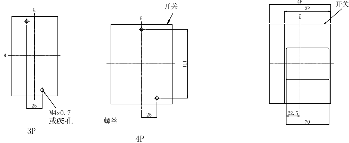
面板开孔尺寸图
