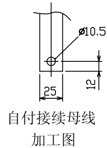
母线最大厚度t8
