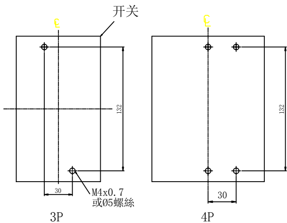
钻孔图
