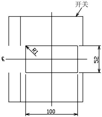
面板尺寸图
