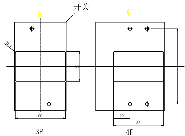
面板尺寸图
