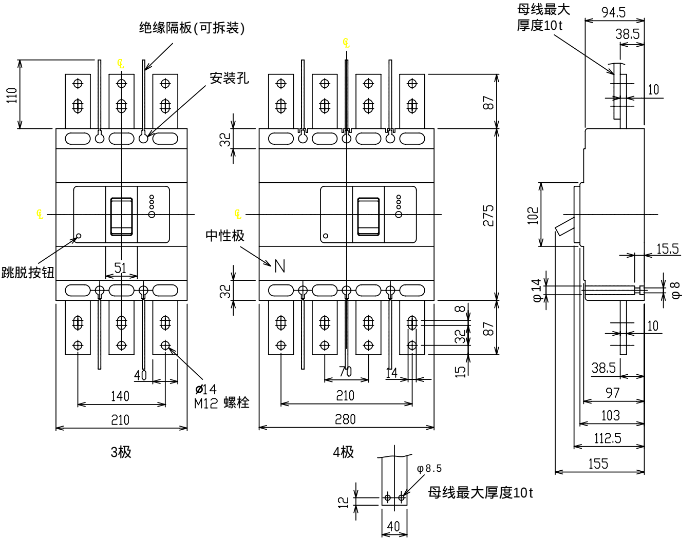
自付接续 母线加工图
