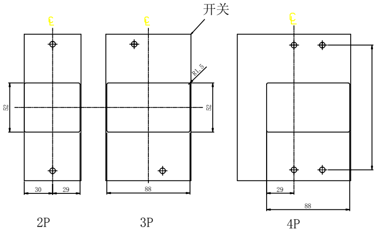
面板尺寸图
