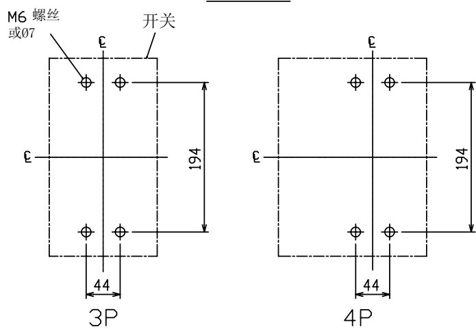
钻孔图
