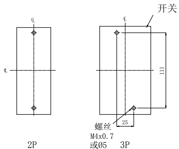
钻孔图
