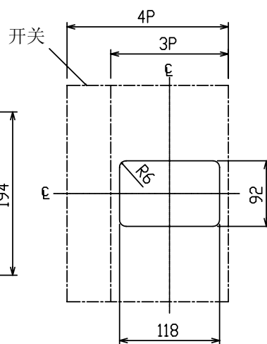
面板孔尺寸图
