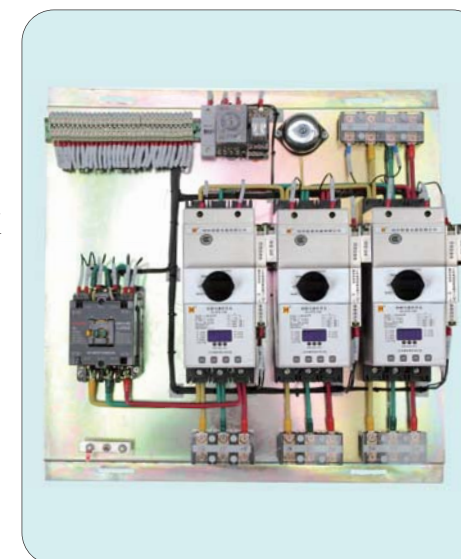
实物底板图
