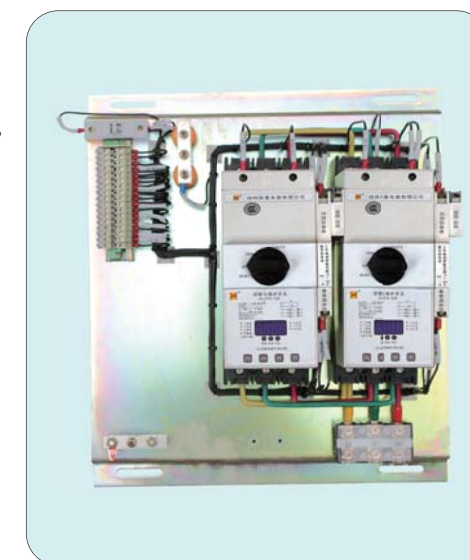
实物底板图
