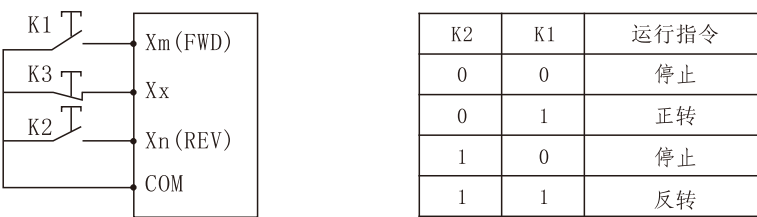
图P7-5 三线式控制模式2示意图
