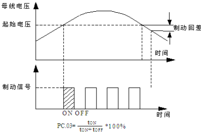
图PC-1能耗制动示意图
