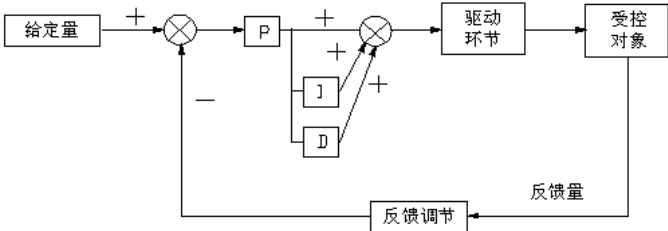
图P8-2 PID调节示意图
