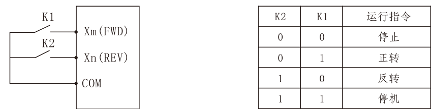
图P7-2 二线式控制模式1示意图
