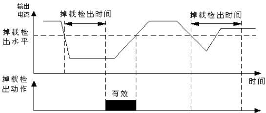
图PA-3 掉载检出示意图
