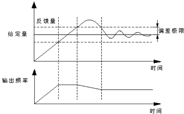
图P8-3偏差极限示意图
