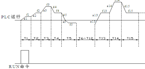
图P9-2 PLC单循环后保持示意图
