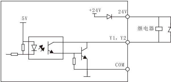
图 3-10 多功能输出端子接线方式
