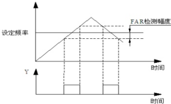
图P7-7 频率到达示意图
