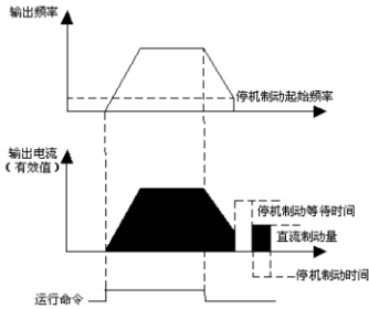
图P1-4 停机直流制动示意图
