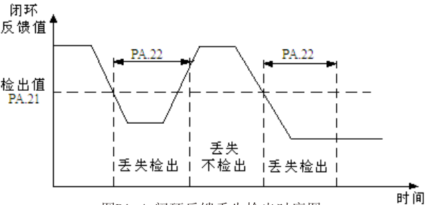
图PA-4 闭环反馈丢失检出时序图
