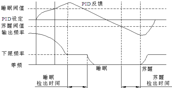
图P8-5 第一种睡眠模式示意图
