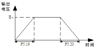
图P5-7 电压控制模式2
