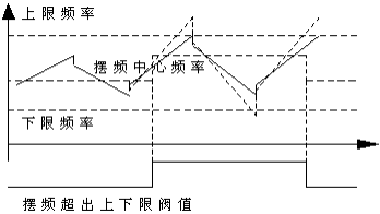
图P7-6 摆频幅度限制示意图
