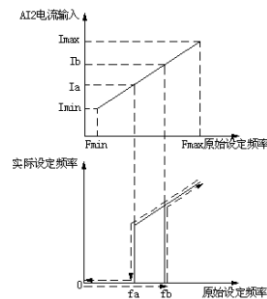
fb：零频运行阈值 fa：fb - 零频回差 图P6-1 零频功能示意图
