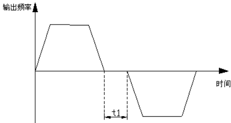
图P1-7 正反转死区时间示意图
