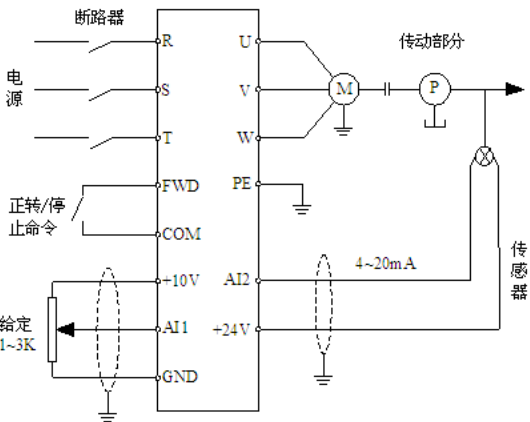
图P8-1 模拟反馈控制系统示意图
