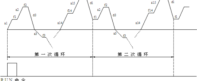
图P9-3 PLC连续循环示意图
