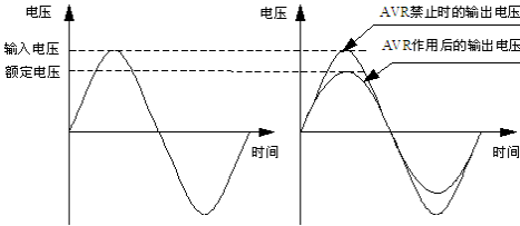
图PC-2 AVR功能示意图
