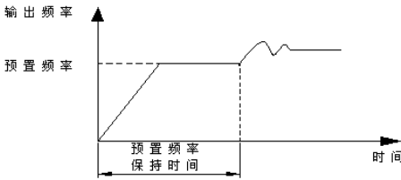
图P8-4闭环预置频率运行示意图
