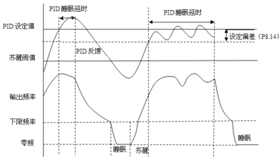
图P8-6 第二种睡眠模式示意图
