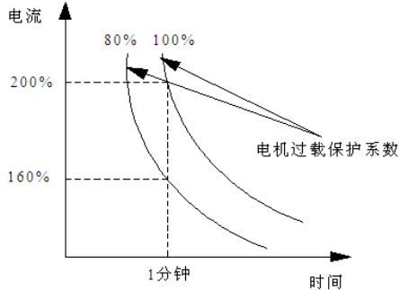
图PA-1 电机过载保护曲线
