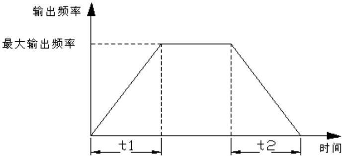
图P0-2 加速时间和减速时间示意图
