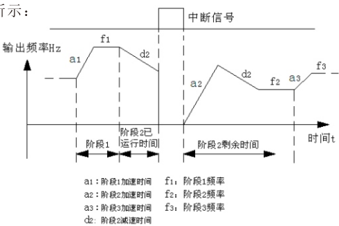
图P9-5 PLC起动方式2
