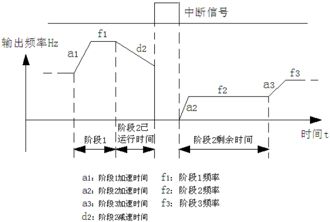
图P9-4 PLC起动方式1
