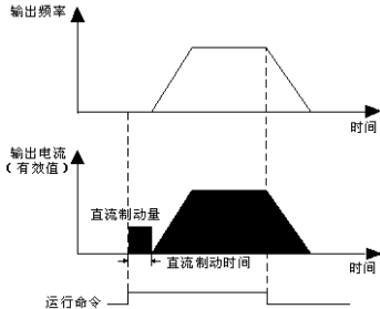
图P1-2 启动直流制动示意图
