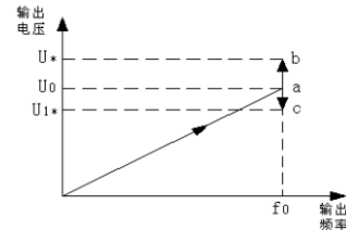
图P5-4 电压控制模式0
