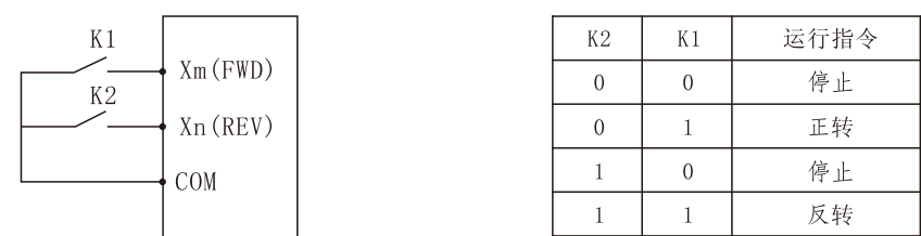
图P7-3 二线式控制模式2示意图
