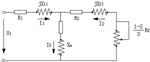
图 P2-1异步电机稳态等效电路图
