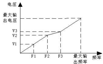
图P5-2 用户设定V/F曲线示意图
