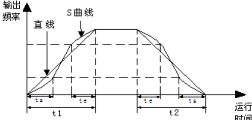
图P1-3 直线与S曲线加减速示意图
