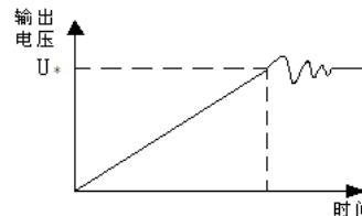
图P5-5 电压控制模式1
