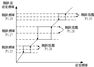
图P1-6 跳跃频率示意图
