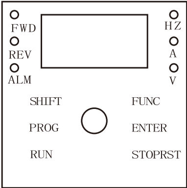
图1-1 9000操作键盘布局图
