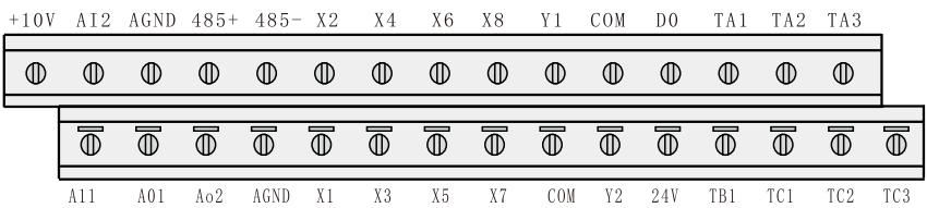
图3-1 0.75KW-2.2KW (G型) 控制回路端子示意图1
