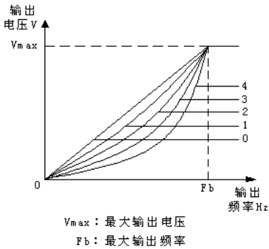
图P5-1 V/F曲线示意图
