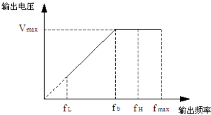
图P0-1 电压与频率示意图
