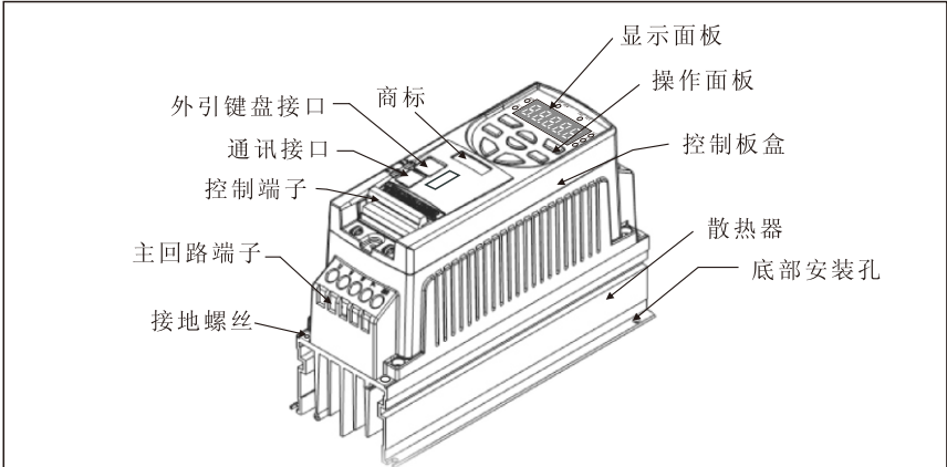
图 2-1 变频器外型图
