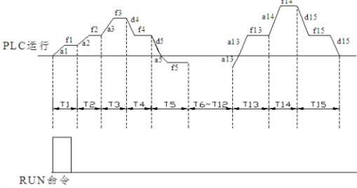
图P9-1 PLC单循环后停机示意图
