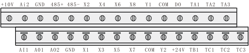
图3-2 2.2KW (C型) 及其以上控制回路端子示意图2
