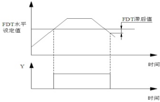
图P7-8 频率水平检测示意图
