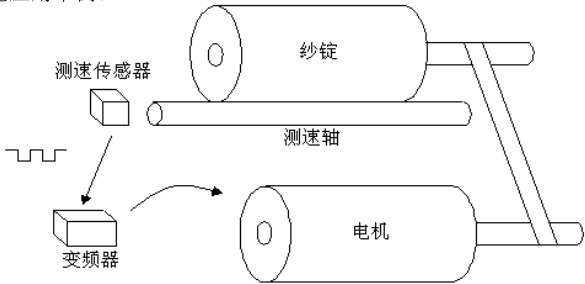
图 P9-7 长停机功能举例图
