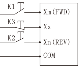
图P7-4 三线式控制模式1示意图
