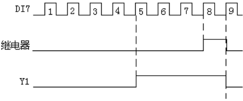
图P7-9 计数器复位设定和计数器检测设定示意图
