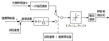
图P4-2 转矩控制简化框图
