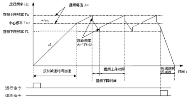
图P9-6 摆频示意图
