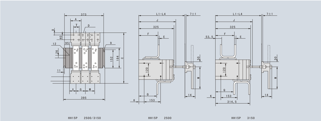
3、HH15P630~3150外形及安装尺寸图
