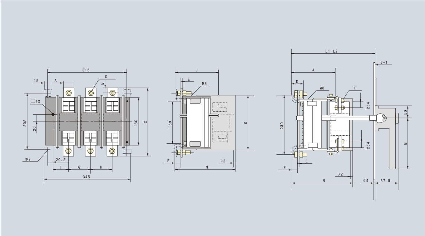
4、HH15隔离开关熔断器组外形及安装尺寸图
