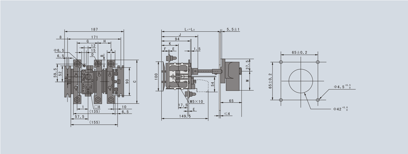
2、HH15P250外形及安装尺寸图
