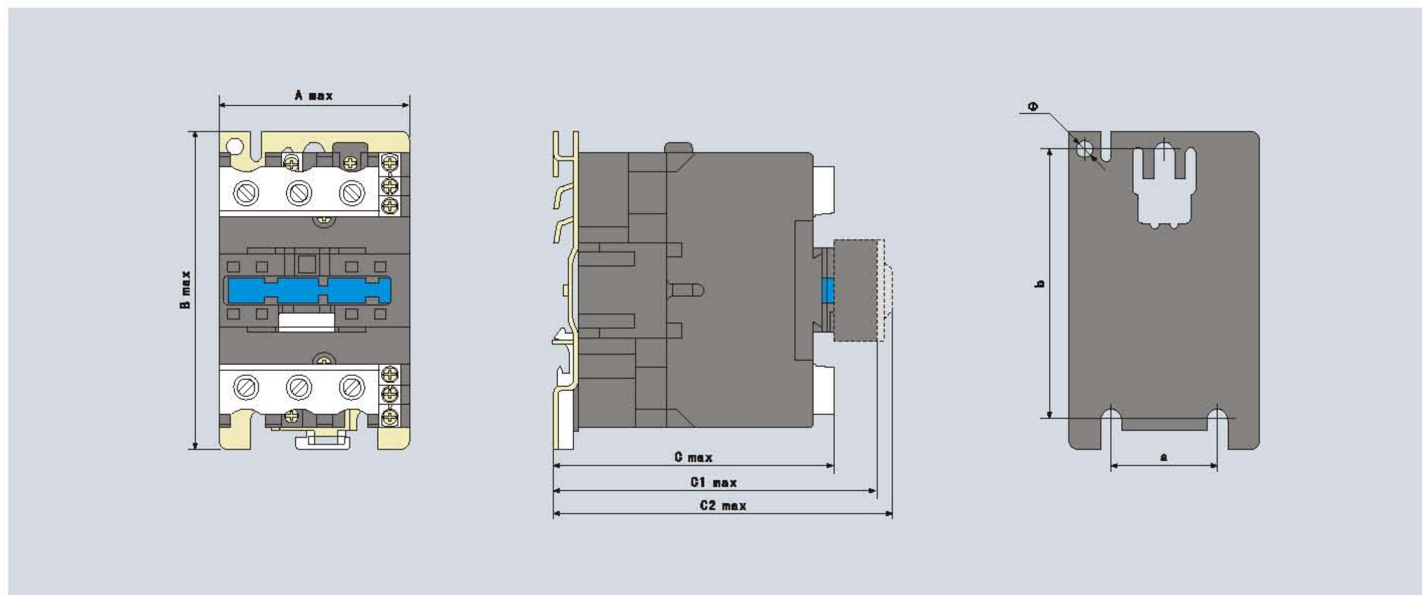
2、CJX2-40~95外形及安装尺寸图
