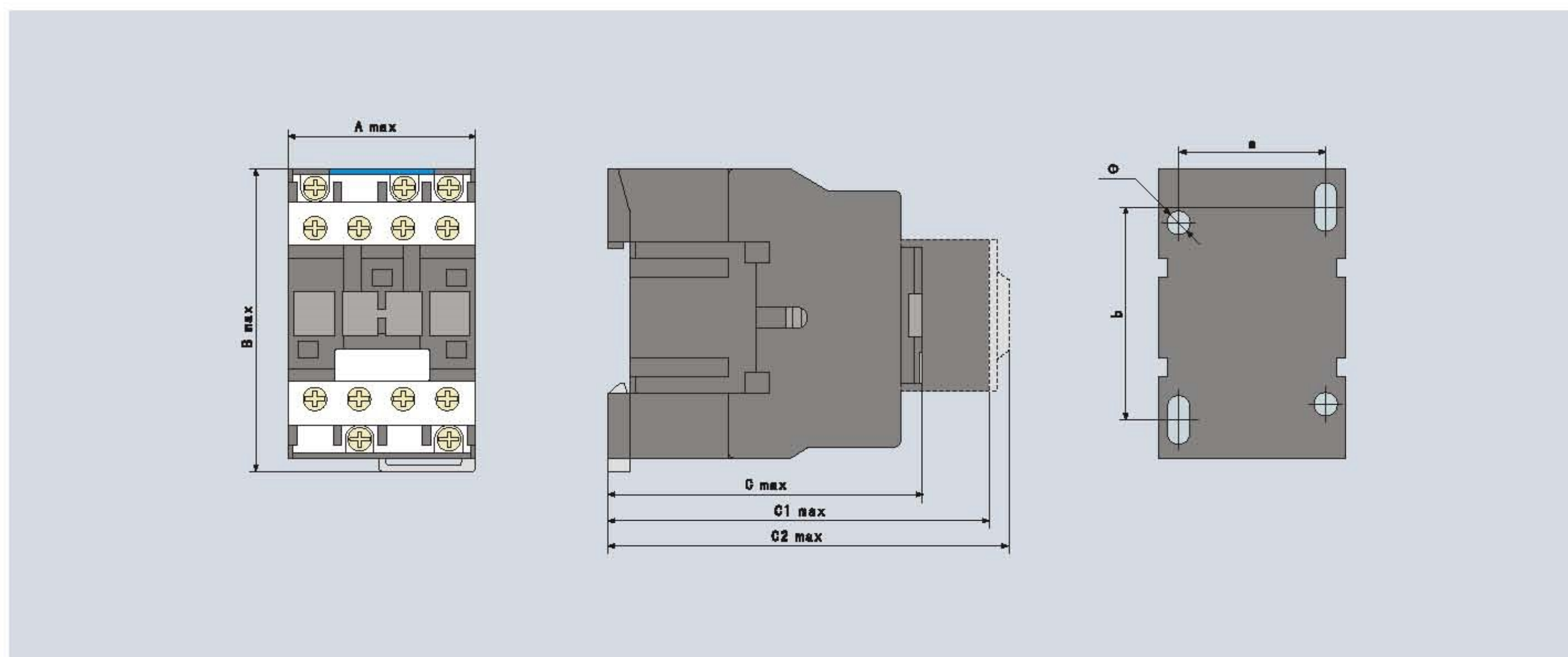
1、CJX2-9~32外形及安装尺寸图
