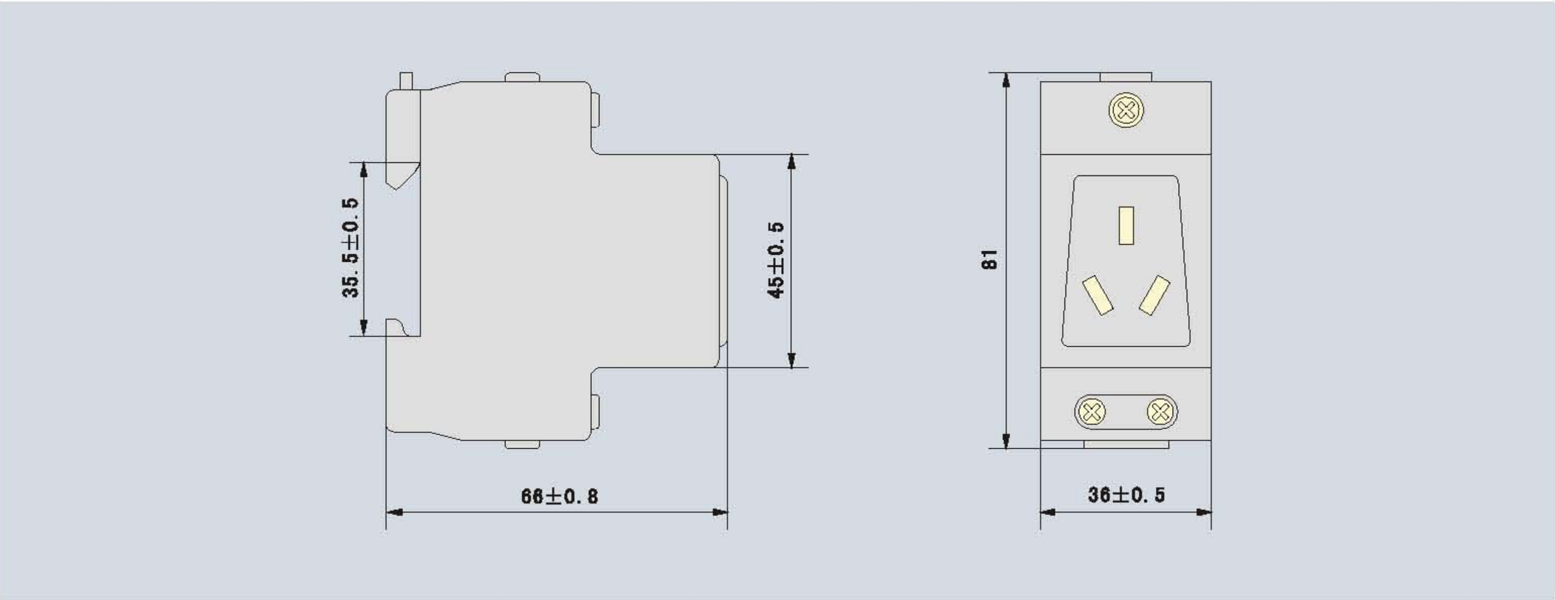
图 2、AC30-10、16/2 250~外形及安装尺寸
