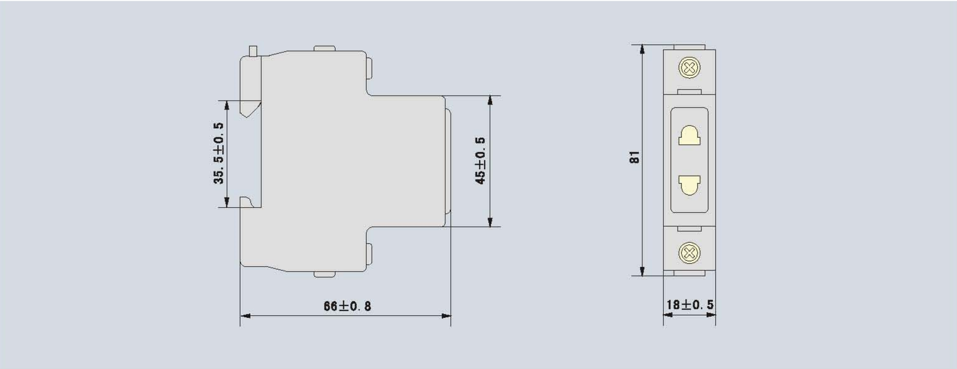
图 1、AC30-10/2 250~外形及安装尺寸
