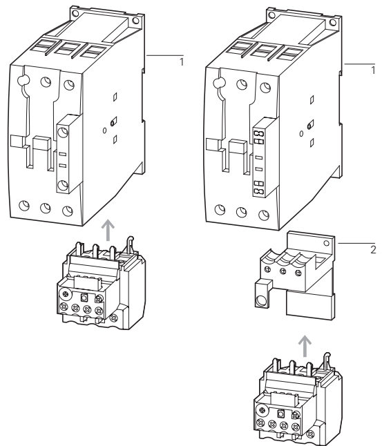
直接安装至接触器
