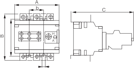
图5 JR20-250, 400, 630
