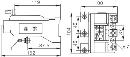
图4 JR20-160
