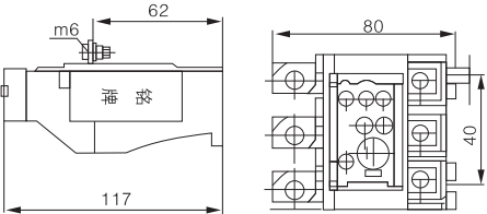
图3 JR20-63
