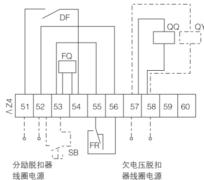
图6 热-电磁式断路器(限流断路器)二次回路接线图
