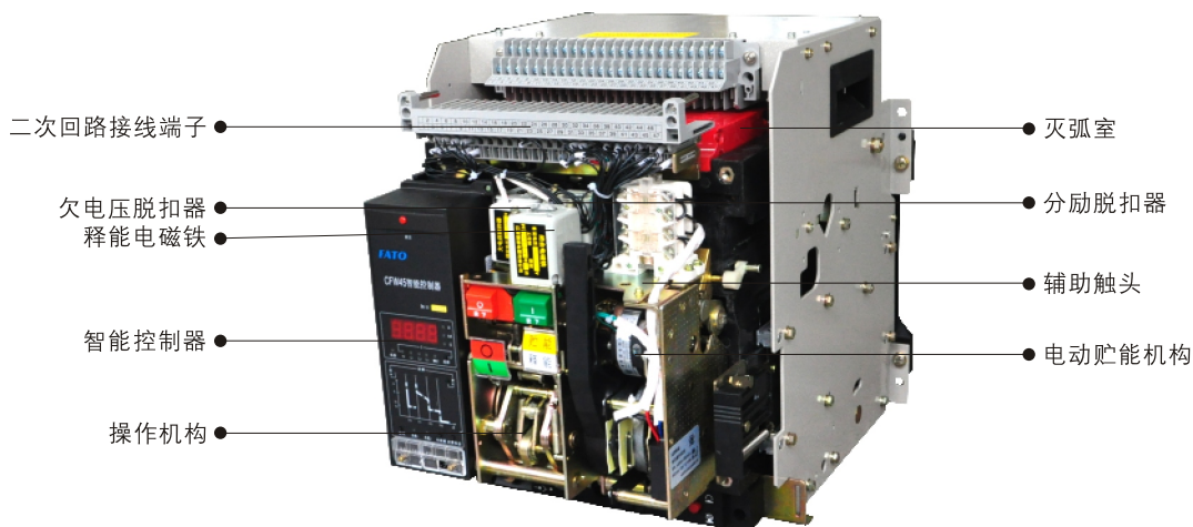
图2-3 CFW45系列智能型万能式断路器抽出位置
