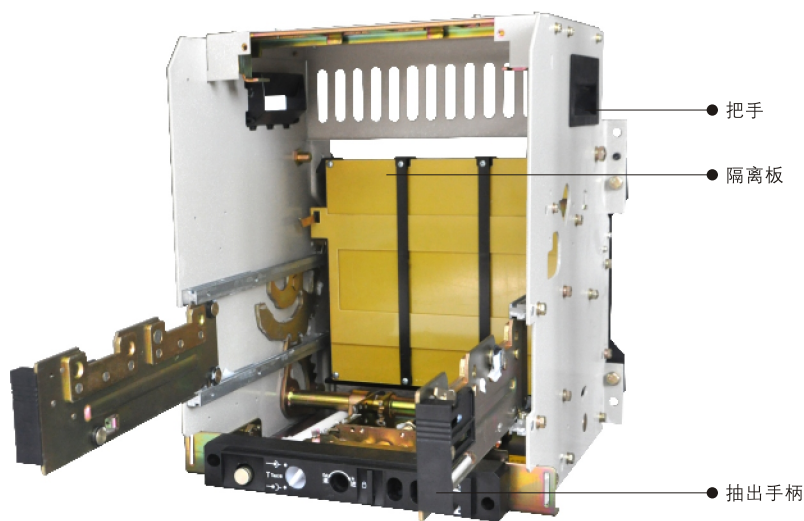
图2-1 CFW45系列智能型万能式断路器
