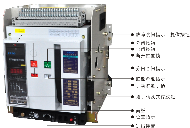
图2-1 CFW45系列智能型万能式断路器
