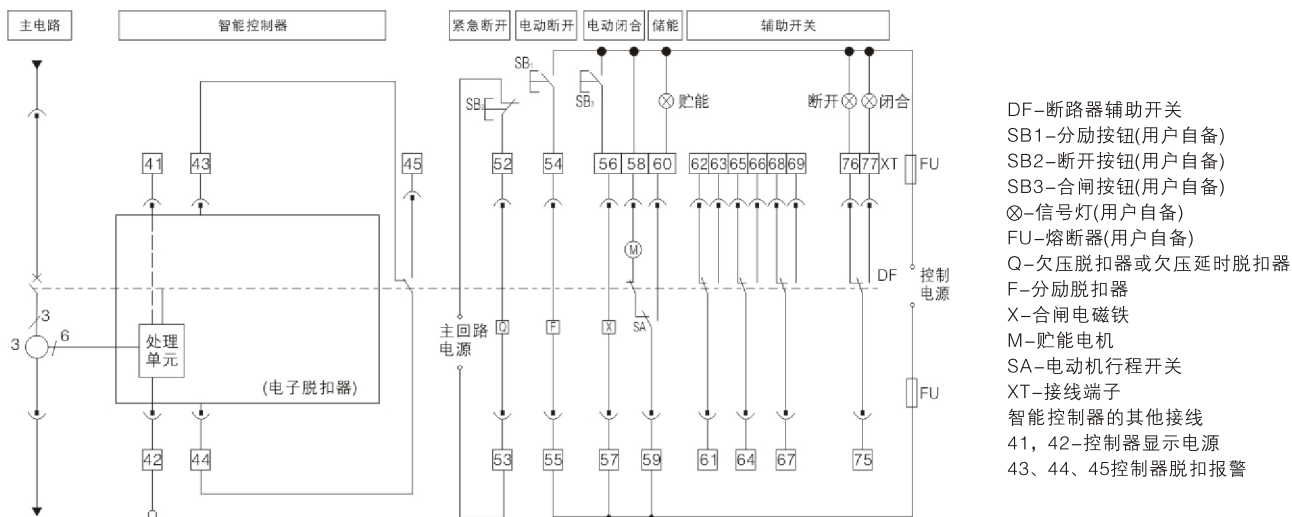
图13a 1000A L,M型智能型万能式断路器二次接线图
