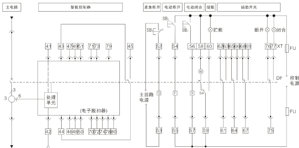
图13b 1000A H型智能型万能式断路器二次接线图
