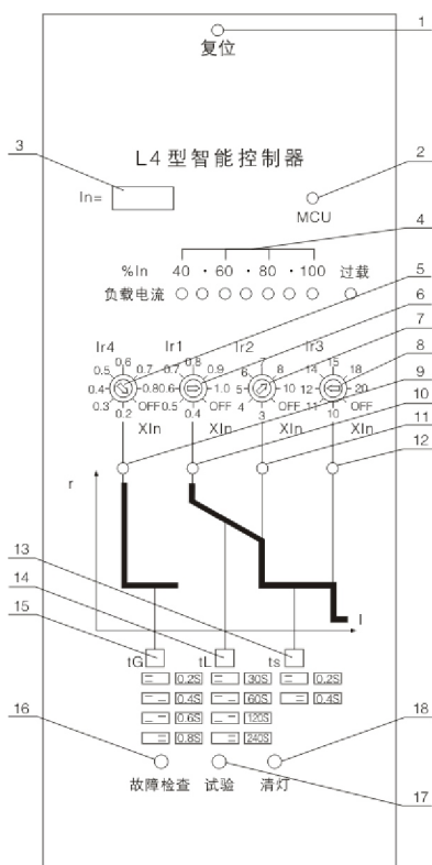
图1-4 面板说明
