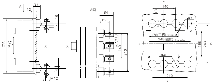
板后接线外形和安装尺寸
