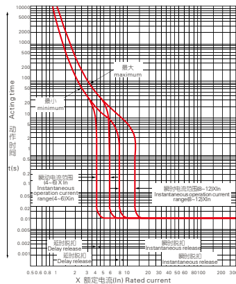
△ GSL1-400时间/电流特性曲线（配电） GSL1-400Time/Current characteristic curve(power distribution)
