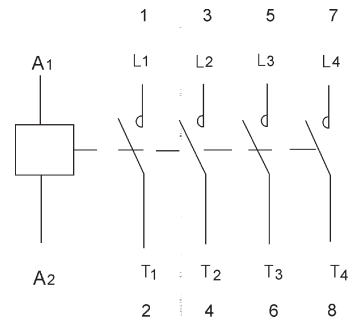
接线图 WIRING PICTURE
