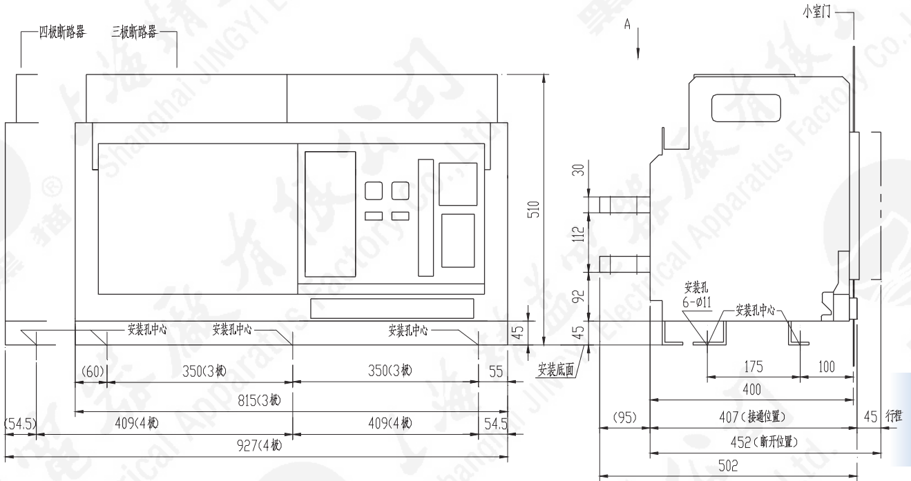
A向 HA3-6300 5000A/3P 标准水平接线端子
