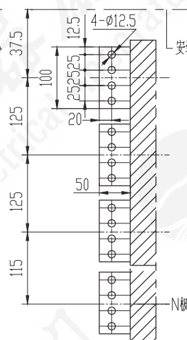
A向 标准水平接线端子 3200A
