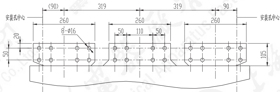
A向 HA3-6300 6300A/3P 标准水平接线端子
