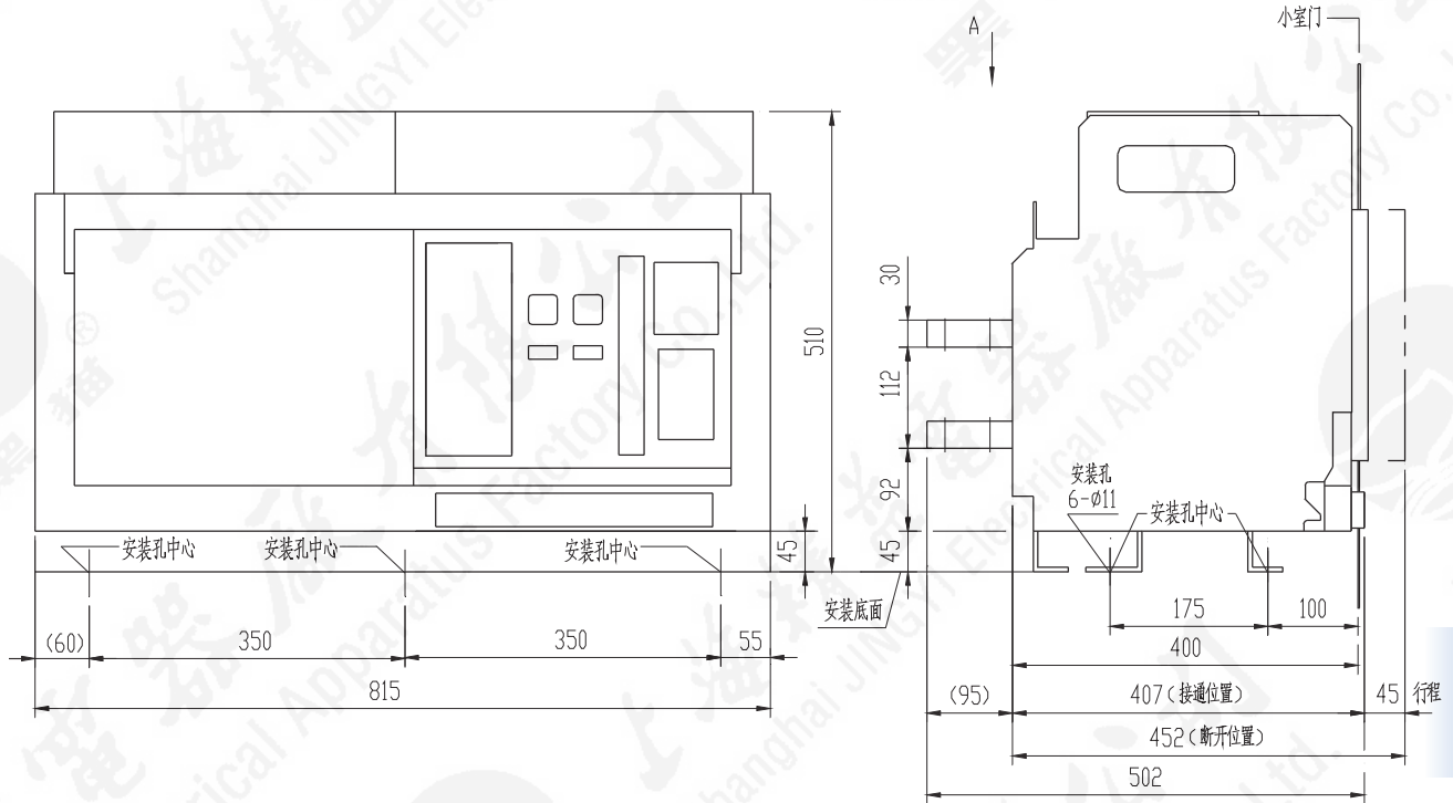
A向 HA3-6300 4000A/3P 标准水平接线端子
