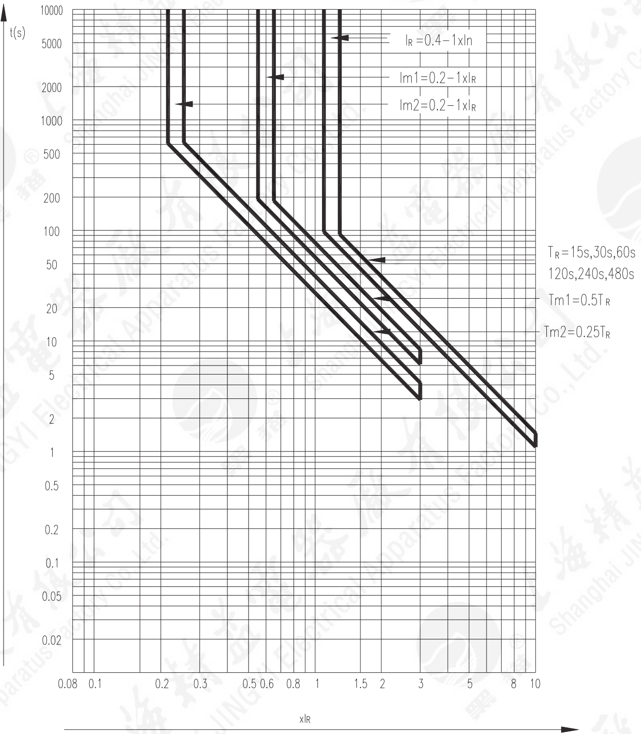
□ 负载监测时间电流特性曲线。
