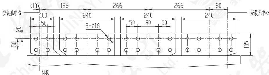
A向 HA3-6300 6300A/4P 标准水平接线端子
