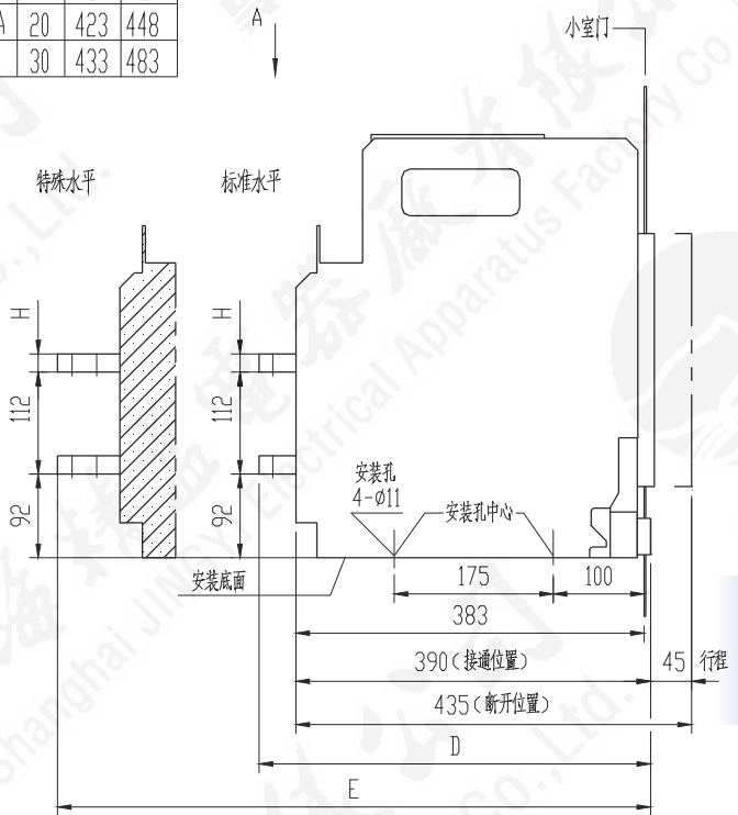
A向 标准水平接线端子 3200A
