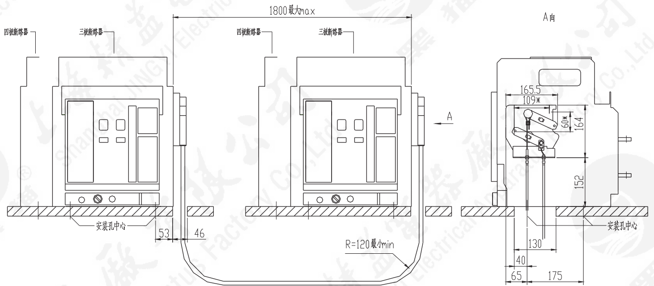
水平安装的两台断路器之间的连接
