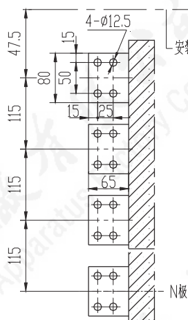
A向 特殊水平接线端子 2000A~2500A
