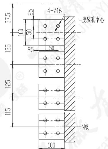
A向 特殊水平接线端子 3200A
