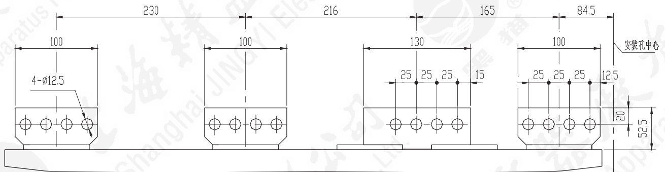
A向 HA3-6300 4000A/4P 标准水平接线端子
