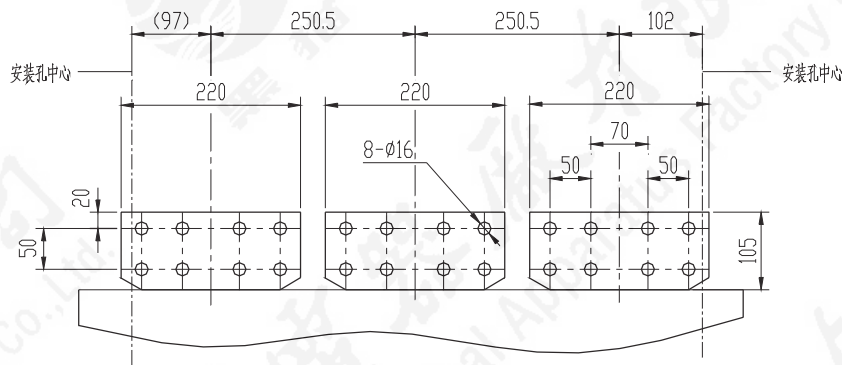
A向 HA3-6300 4000A/4P 标准水平接线端子
