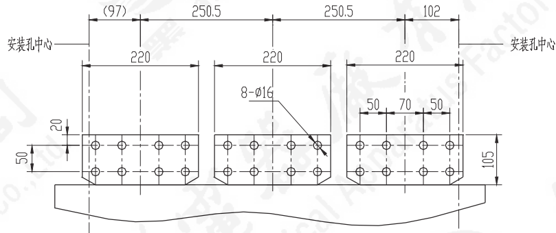
A向 HA3-6300 5000A/3P 标准水平接线端子
