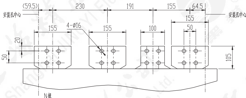
A向 HA3-6300 4000A/4P 标准水平接线端子
