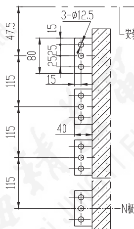
A向 标准水平接线端子 2000A~2500A
