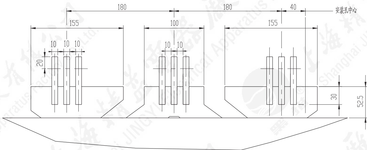
A向 十字垂直线端子
