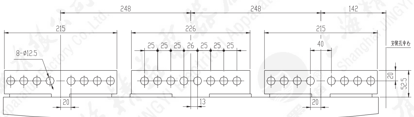
A向 HA3-6300 5000A/3P 标准水平接线端子
