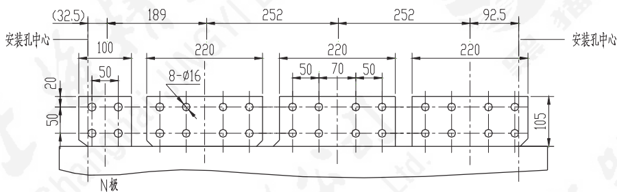
A向 HA3-6300 5000A/4P 标准水平接线端子
