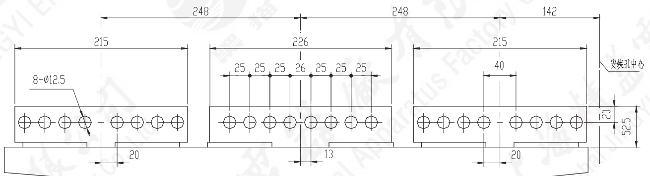
A向 HA3-6300 4000A/4P 标准水平接线端子
