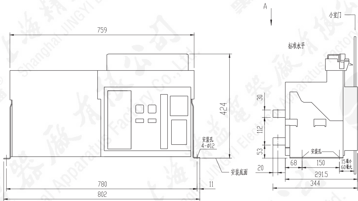
A向 HA3-6300 4000A/3P 标准水平接线端子
