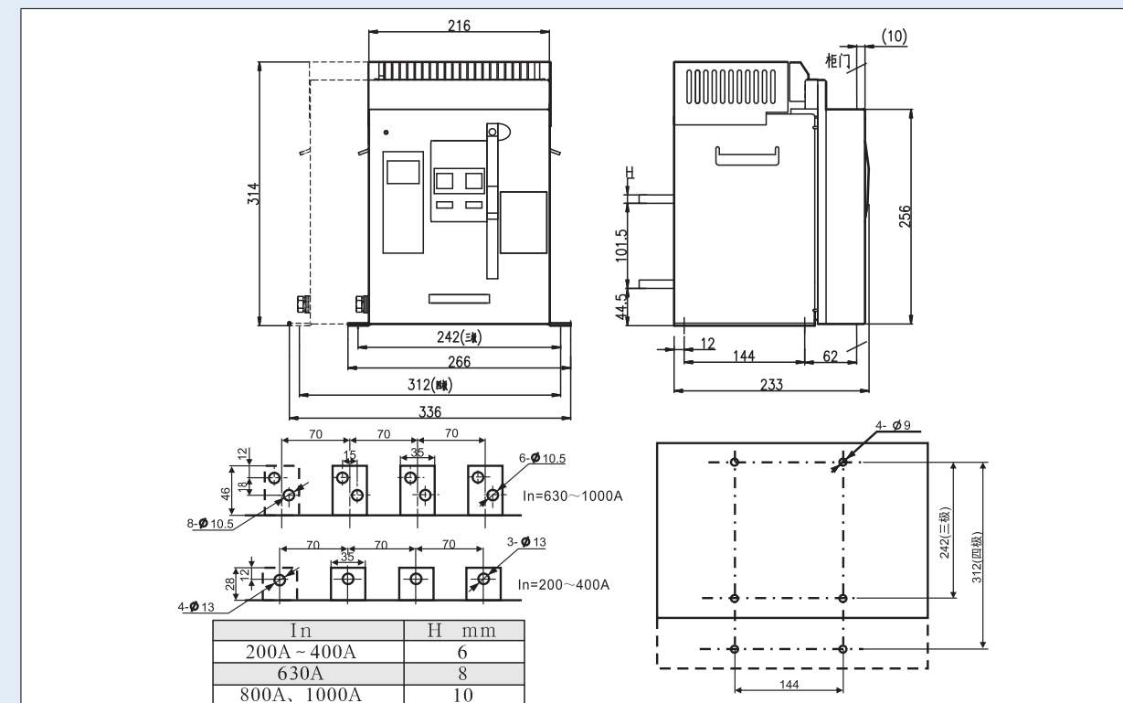
图8 固定式断路器安装尺寸及外形尺寸（HSW1-1000，HSW1-1000/4）
