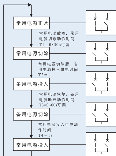
电网-电网型自投自复功能逻辑图
