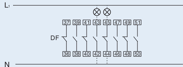
图6 (辅助开关为四常开四常闭单独接线，仅针对Inm=2000及以上壳架官兵器器)
