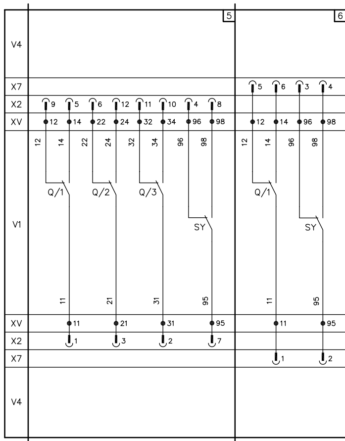
图 (5) 3 个断路器分闸 / 合闸的电气信号转换触头和 1 个由于热磁脱扣器、SOR-C 或 UVR-C 或测试按钮动作使断路器脱扣的电气信号转换触头 (3Q + 1SY)
