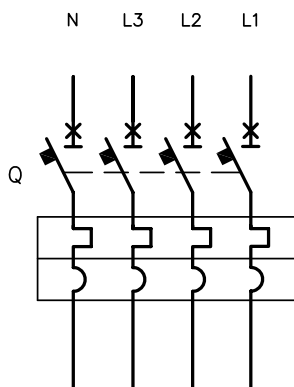
带热磁脱扣器的 4 极断路器
