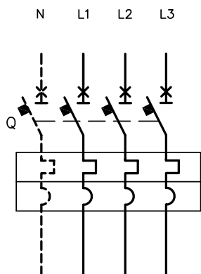
带热磁脱扣器的 3 极断路器
