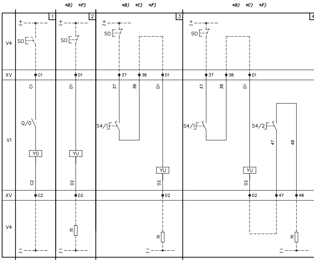
图 (1) 分励脱扣器 (SOR-C 或 YO) 图 (2) 欠电压脱扣器 (UVR-C 或 YU) 图 (3) 瞬时欠压脱扣器带 1 个串联触头 (AUE-C + UVR-C) 图 (4) 瞬时欠压脱扣器带 2 个串联触头 (AUE-C + UVR-C)
