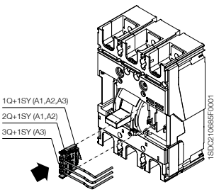
3 极断路器
