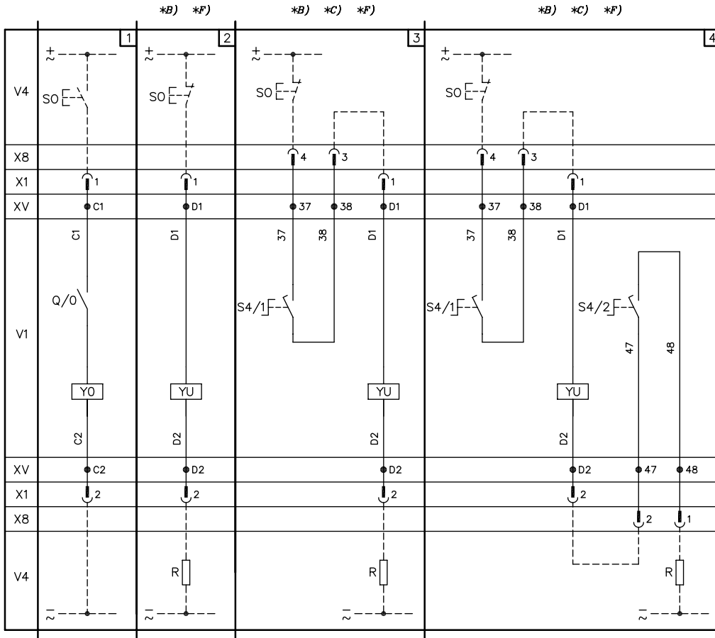
图 (1) 分励脱扣器 (SOR-C 或 YO) 图 (2) 欠电压脱扣器 (UVR-C 或 YU) 图 (3) 瞬时欠电压脱扣器带 1 个串联触头 (AUE-C + UVR-C) 图 (4) 瞬时欠电压脱扣器带 2 个串联触头 (AUE-C + UVR-C)
