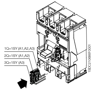
4 极断路器
