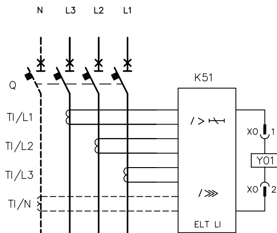
带电子脱扣器的 3 极断路器
