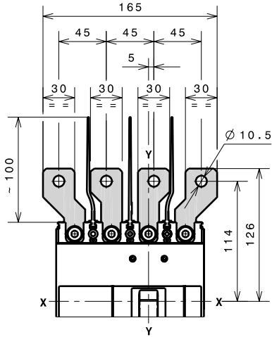
4 极
