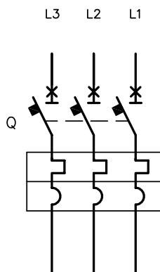
带热磁脱扣器的 3 极断路器
