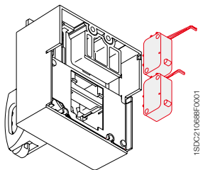
预先动作辅助触头
