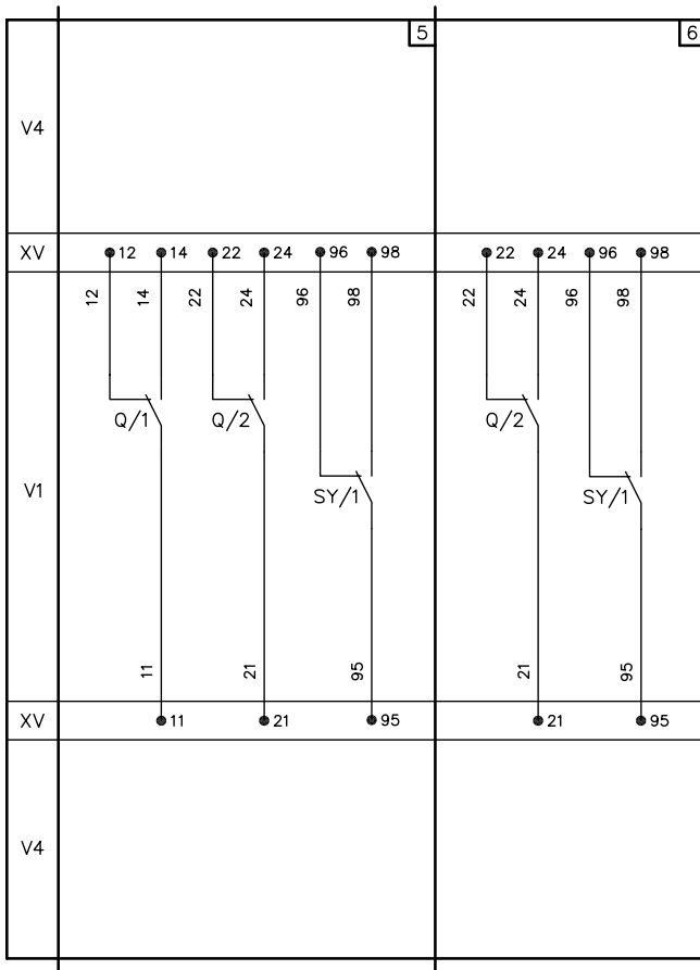
图 (5) 2 个断路器分闸 / 合闸的电气信号转换触头和 1 个由于热磁脱扣器、SOR-C 或 UVR-C 或测试按钮动作使断路器脱扣的电气信号转换触头 (2Q + 1SY)
