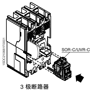
3 极断路器
