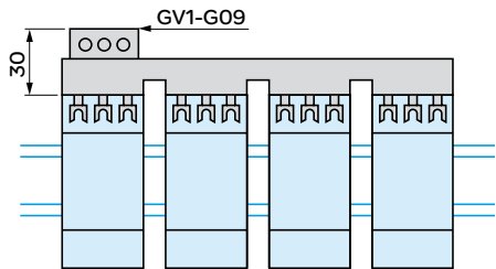
带接线端子模块 GV1-G09
