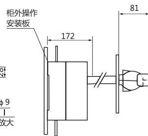
柜外操作安装底板
