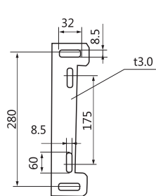
柜外操作安装底板
