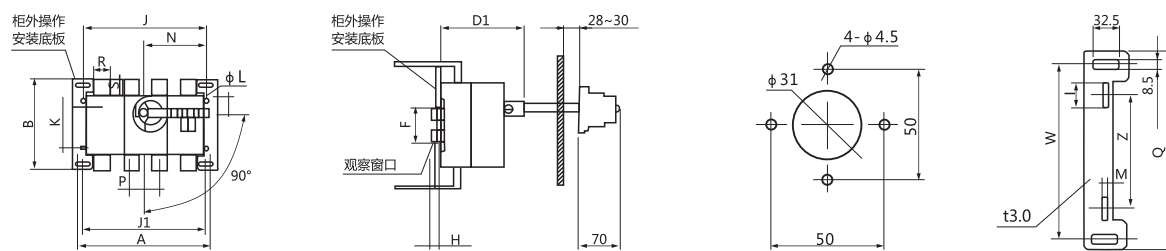
RDH5(HGL)Z-125A~630A/BJK柜外操作
