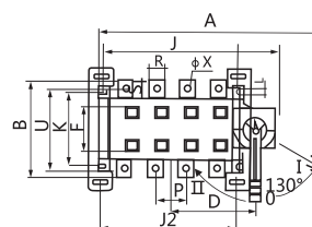
RDH5(HGL)Z-125~630A/J
