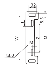
RDH5(HGL)Z-125~630A/J
