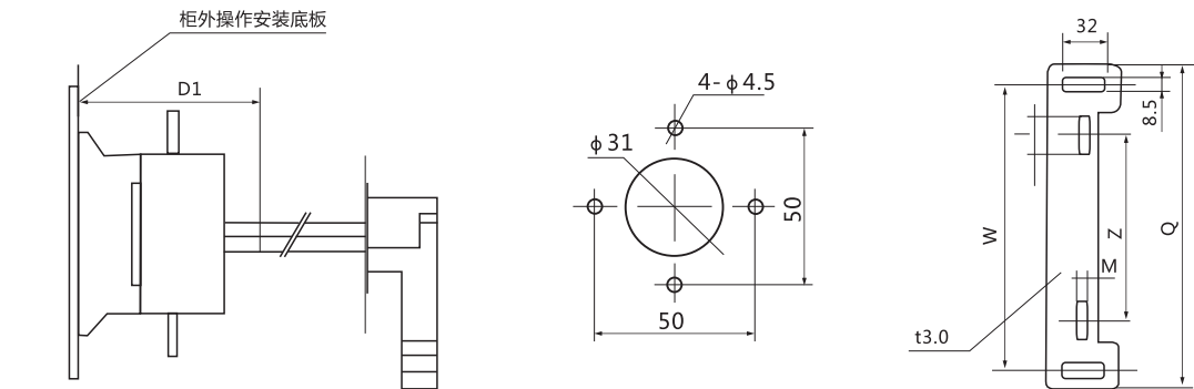
柜外手柄座安装尺寸
