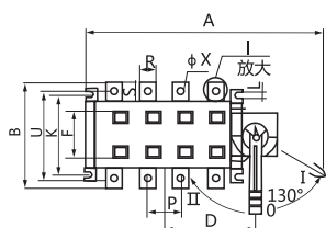
RDH5(HGL)Z-125~630A
