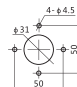
B型柜外手柄
