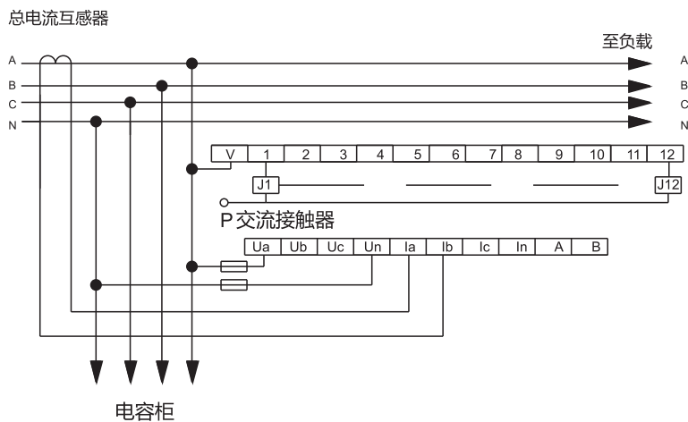
图4 JKG2B(JKW5B)接线图(取样电压220V) 开孔尺寸：162X102 ( mm )
