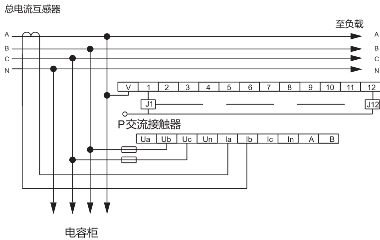
图3 JKG2B(JKW5B)接线图(取样电压380V)
