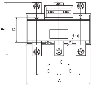
图1 HD11F-200~1600/38
