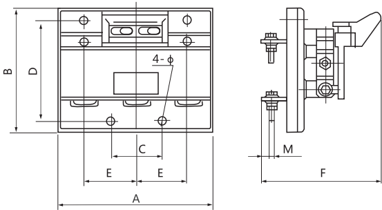
图2 HD11F-200~1000/39
