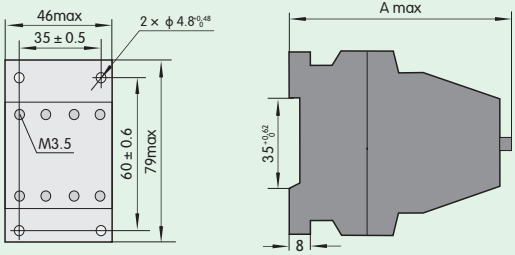
图2 JZC1-□□/Z系列
