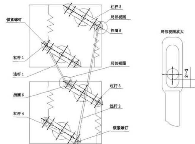
两台断路器之间的硬杆联接示意图。
