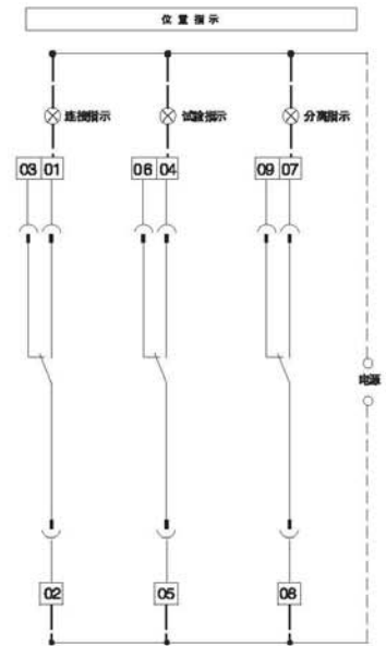
抽屉三位电气指示接线示意图。
