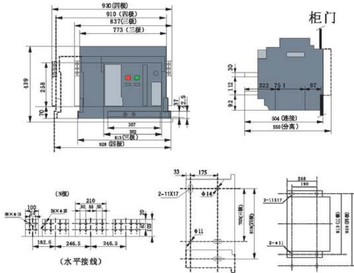
19.6 TGW45-6300 (In=4000-5000A) 抽屉式断路器外形尺寸与安装尺寸图。
