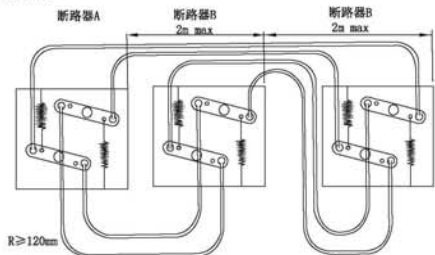
三台断路器的软杆联锁
