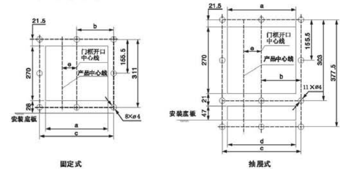
19.8 面板开孔安装尺寸图。
