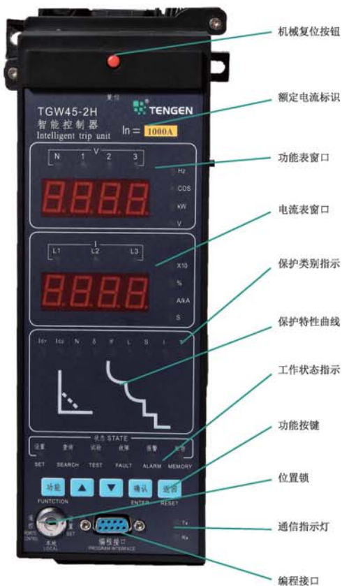
控制器面板区域图
