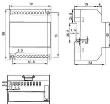
ST 电源模块 (IV)
