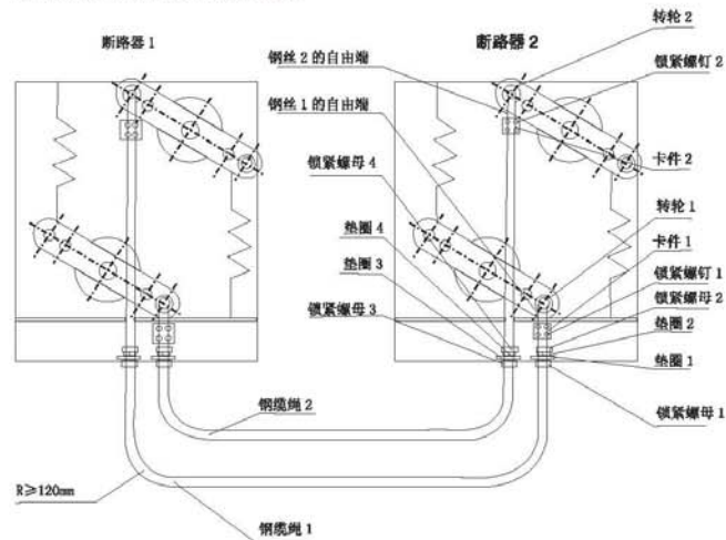
两台断路器之间的钢丝绳联接示意图。
