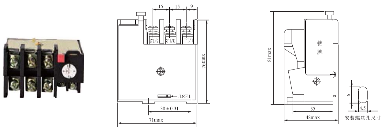
图1 TGR36-32独立式安装
