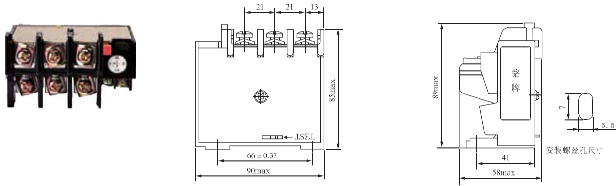
图2 TGR36-63独立式安装
